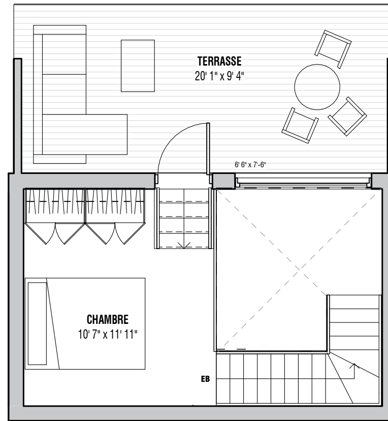
NIVEAU MEZZ.
