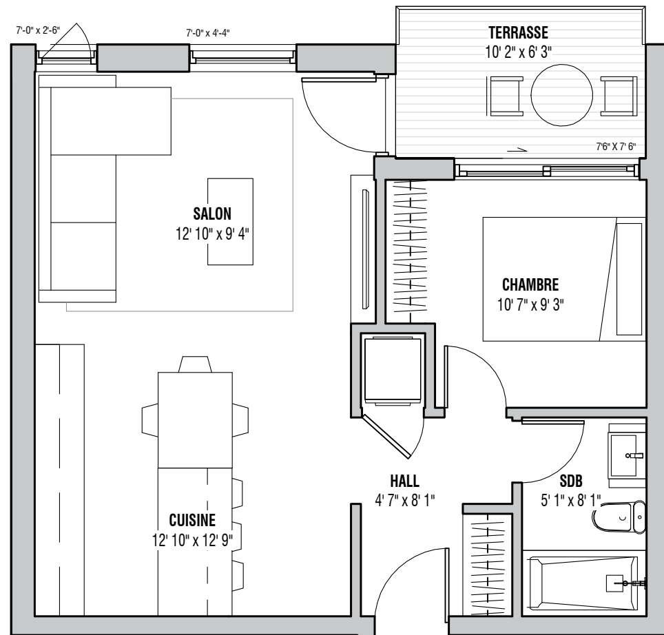
NIVEAU 02
